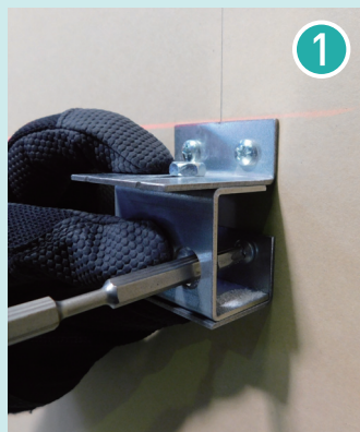
壁下地に対し廊下用支持金具をビス固定
