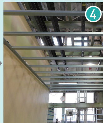
DHメインの通りを調整し下地組み完了
